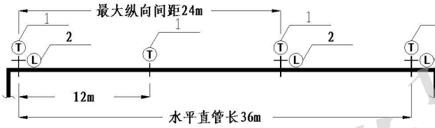
图 21 水平直管段纵向抗震支吊架设置示意 1—抗震支吊架;2—纵向抗震支吊架
