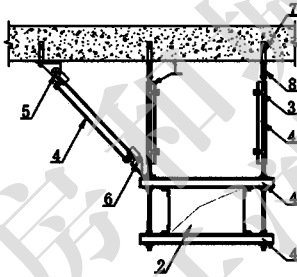
图1 抗震支吊架示意图
