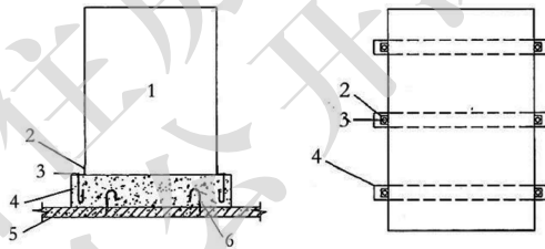
图 16 给水水箱、水箱基础与楼板或底板连接示意
