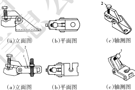
图2 抗震连构件示意图
