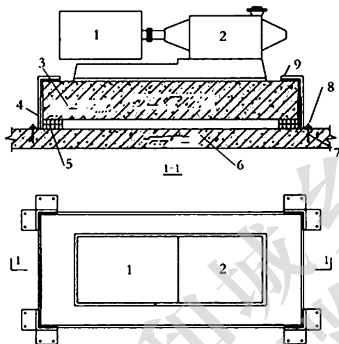
图 18 水泵限位器布置
