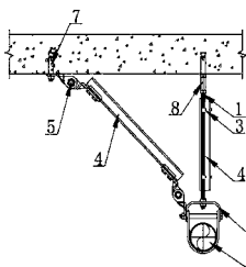
图 3 侧向抗震支吊架示意图
