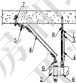
图 4 纵向抗震支吊架示意图
