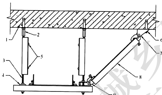
图 6 门型抗震支吊架示意图
