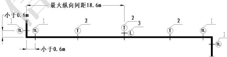
图 23 水平管线转弯时抗震支吊架设置示意 1—侧向抗震支吊架;2—抗震支吊架;3—纵向抗震支吊架
