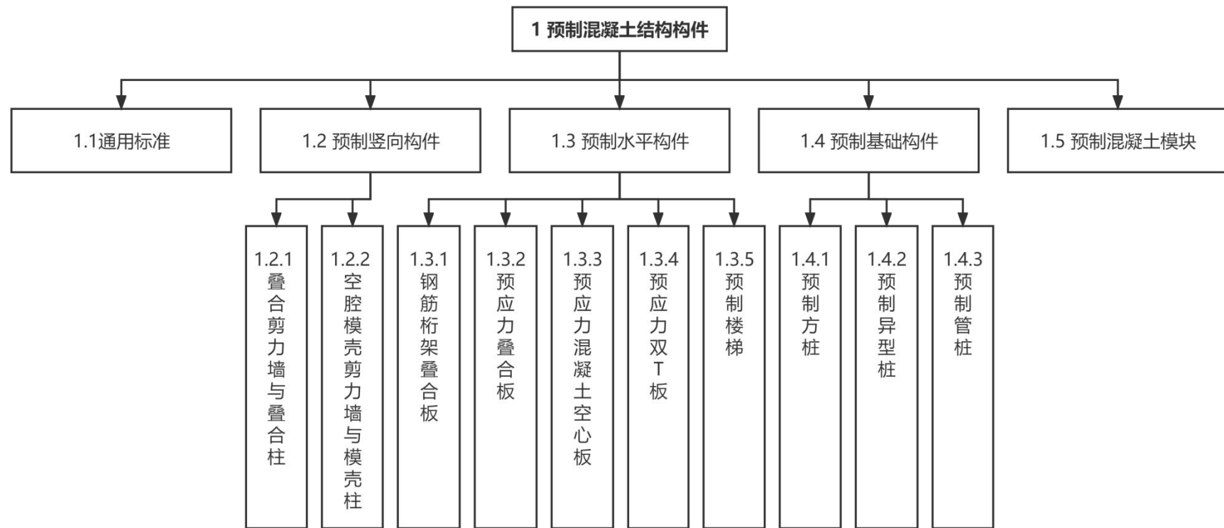
图2 预制混凝土结构构件质量标准体系框架
