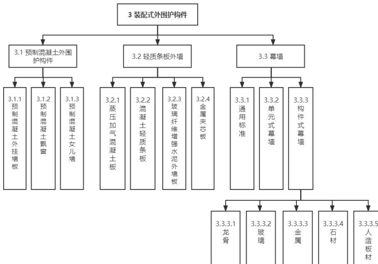
图 4 装配式外围护构件质量标准体系框架
