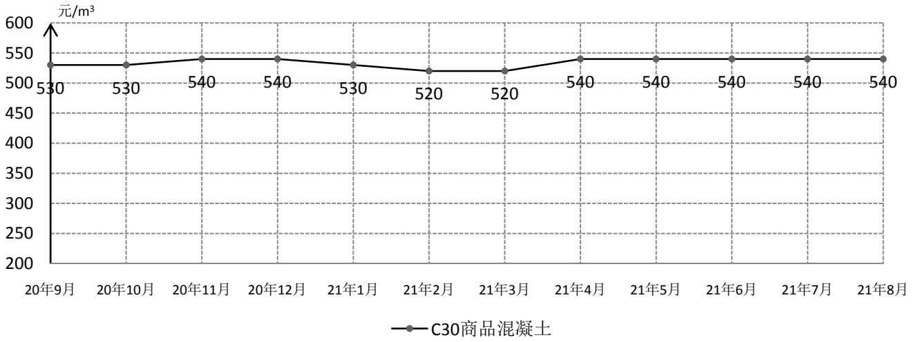
近期海口地区部分主要材料价格走势
